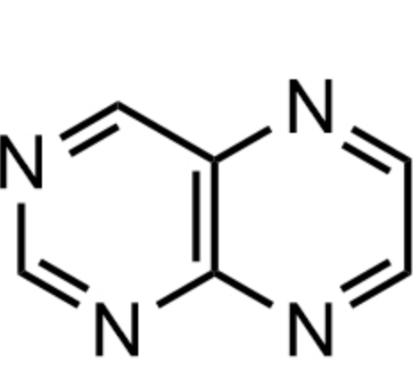
pteridine 蝶啶
