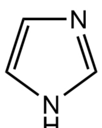
Imidazole 咪唑
