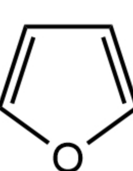
Furan 呋喃
