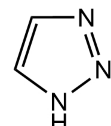
1,2,3-Triazole 三唑
