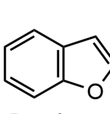
Benzofuran 氧茚/香豆酮
