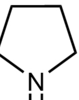
Pyrrolidine 吡咯烷
