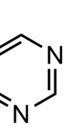
Pyrimidine 嘧啶
