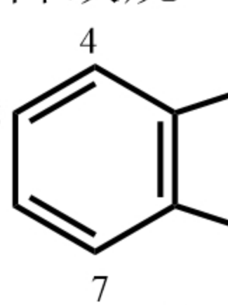
Indene 茚
