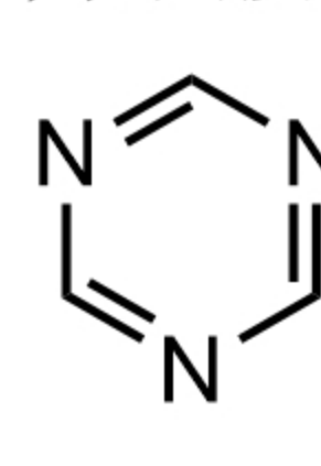
1,3,5-Triazine 三嗪
