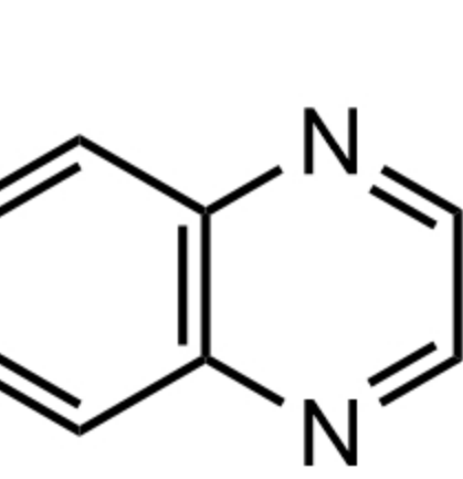
Quinoxaline 喹喔啉
