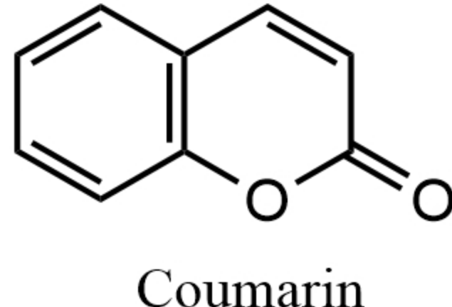
Coumarin 香豆
