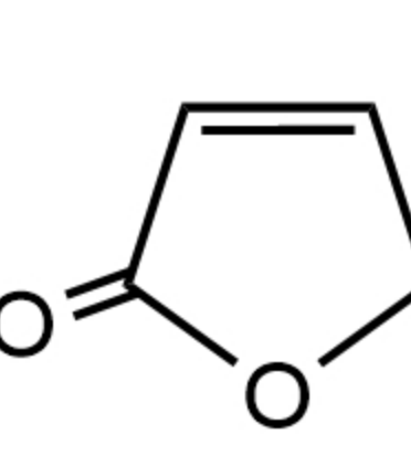
Maleic anhydride 顺丁烯二酸酐
