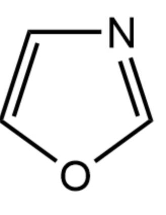
Oxazole 恶唑
