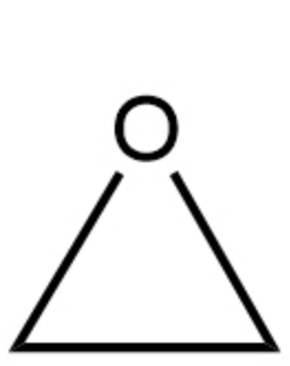
Oxirane 环氧乙烷
