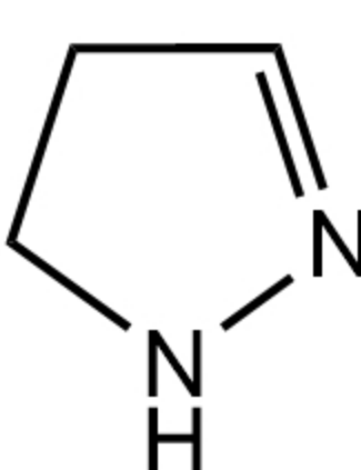
2-Pyrazoline 吡唑琳
