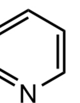
Pyridine 吡啶
