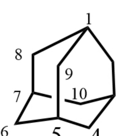
Admantane 金刚烷
