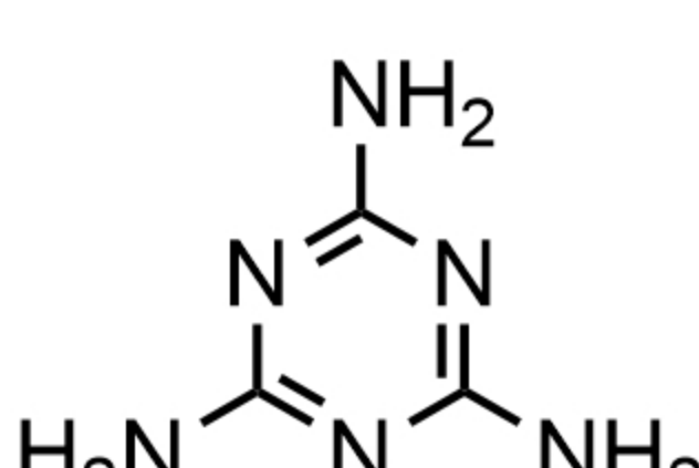
triaminometriazine 三氨基均三嗪
