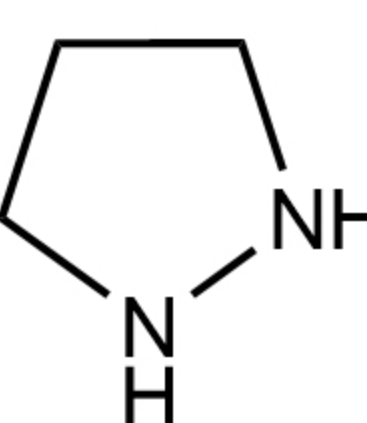
Pyrazolidine 吡唑烷
