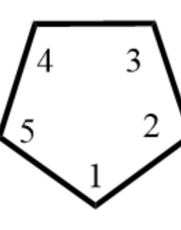
Cyclopentane 环戊烷
