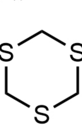
1,3,5-Trithiane 三噻烷
