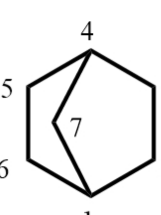
Norbornane 降莰烷
