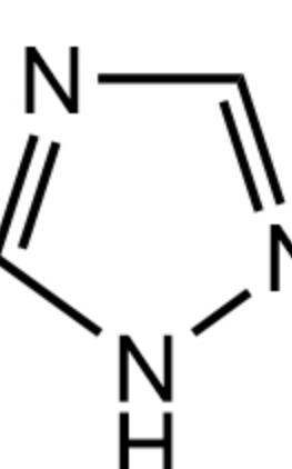
1,2,4-Triazole 三唑
