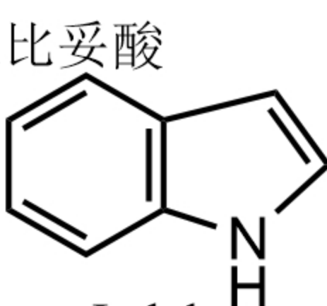
Indole 吲哚
