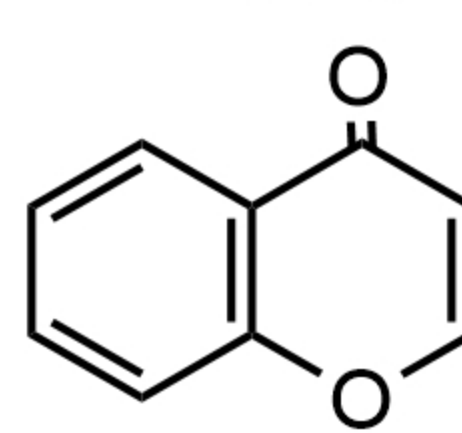
Benzogamapyranone 苯并伽马吡喃酮
