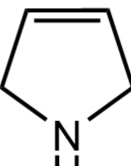
3-pyrroline 吡咯琳
