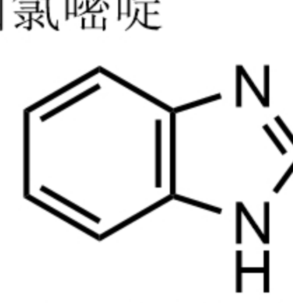
Benzimidazole 苯并咪唑
