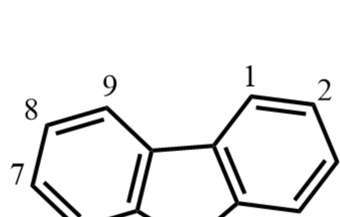
Dibenzofuran, 氧芴
