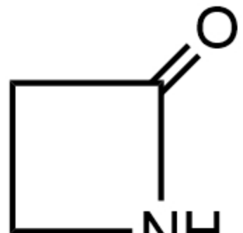
beta propionactam beta-丙内酰胺
