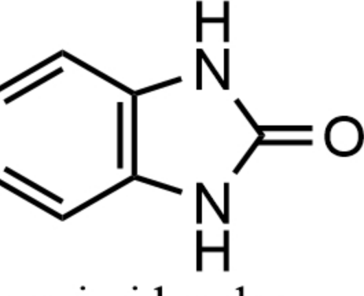
benzimidazolone 苯并咪唑酮
