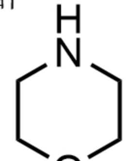
Morpholine 吗啉
