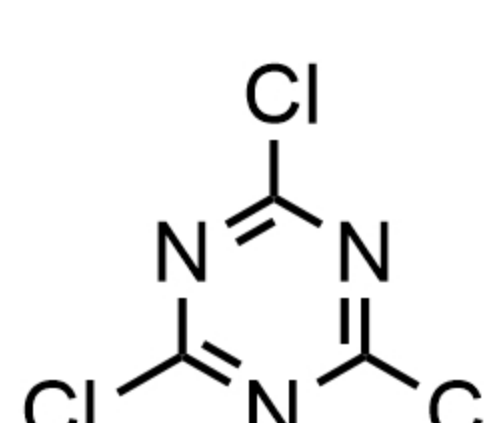
trichlorometriazine 三氯均三嗪
