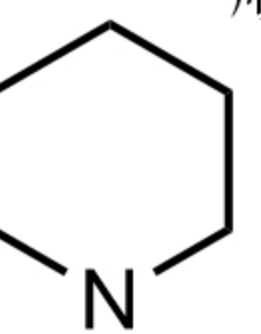
Piperidine 哌啶
