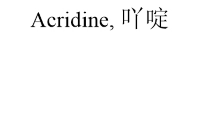
Acridine, 吖啶
