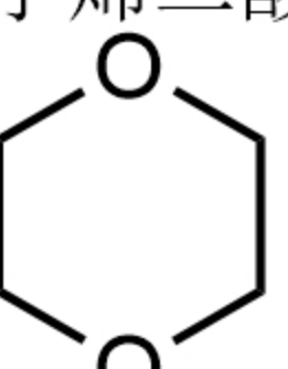
1,4-Dioxane 二氧己环
