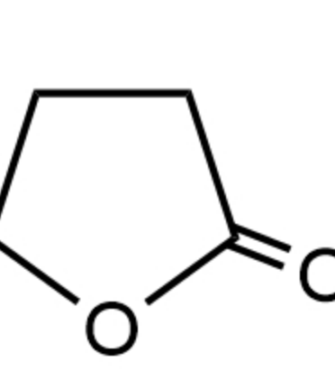
butyrolactone gama-丁内酯
