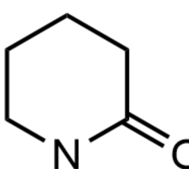
caprolactam 己内酰胺
