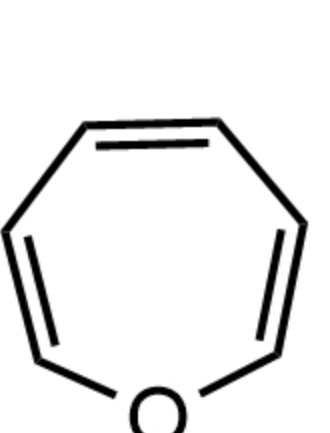
oxapine 氧杂莰
