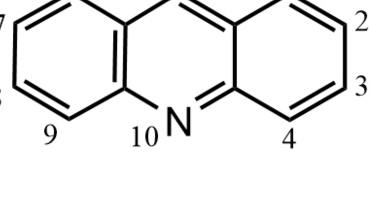
Acridine, 吖啶
