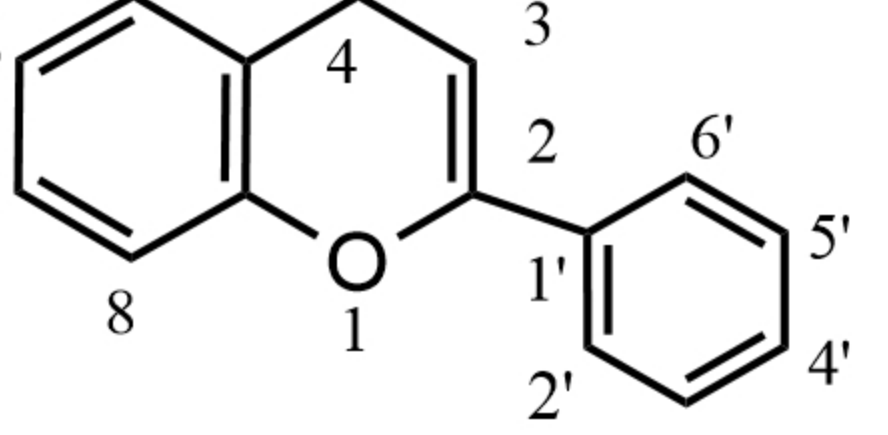
Flavone, 黄酮
