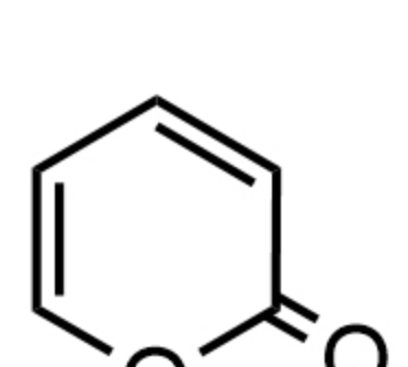
Alpha pyranone 阿尔法-吡喃酮
