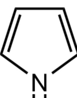
Pyrrole 吡咯
