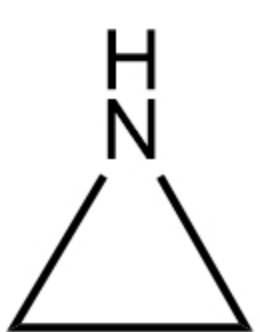
Aziridine 吖丙啶
