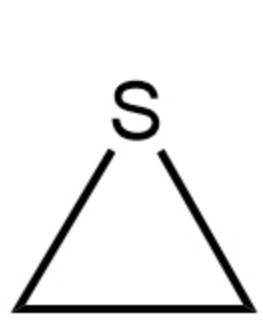
Thiirane 环硫乙烷
