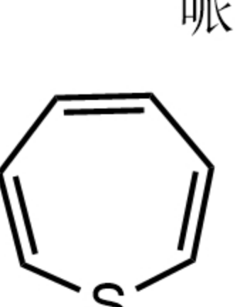
thiazepine 硫杂莰
